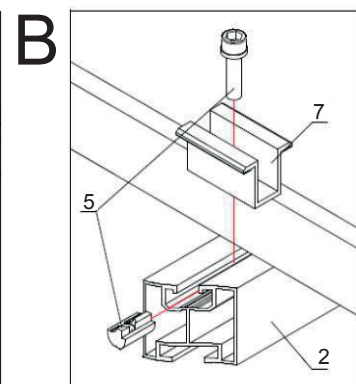
Moduļu uzstādīšana
