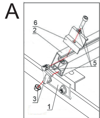
Profilu uzstādīšana
