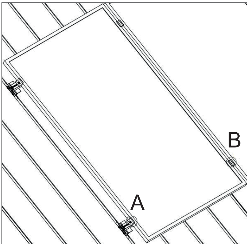
Profilu savienošana
